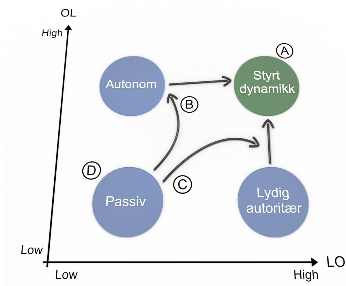
Figur 9: Dynamisk modell
