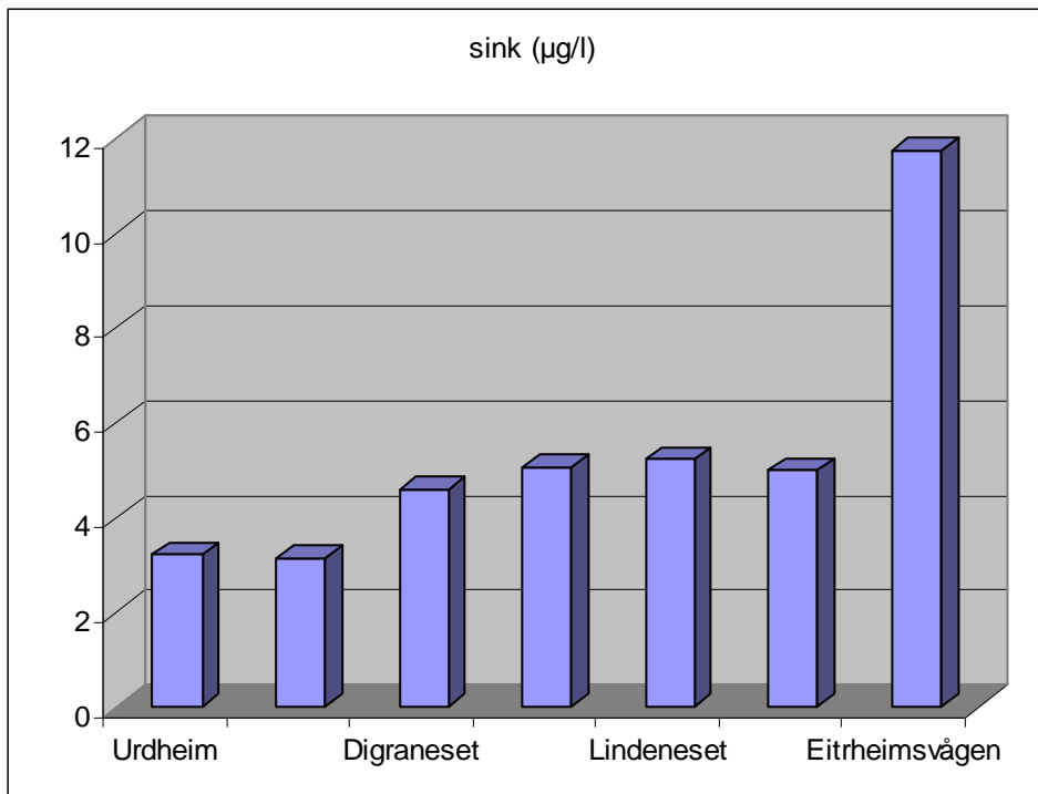
Figur 6. Årsgjennomsnittet av sink ( \mu\text{g/l} ) i overflatevann fra innerst (høyre) til ytterst (venstre) i Sjørfjorden 2009.
