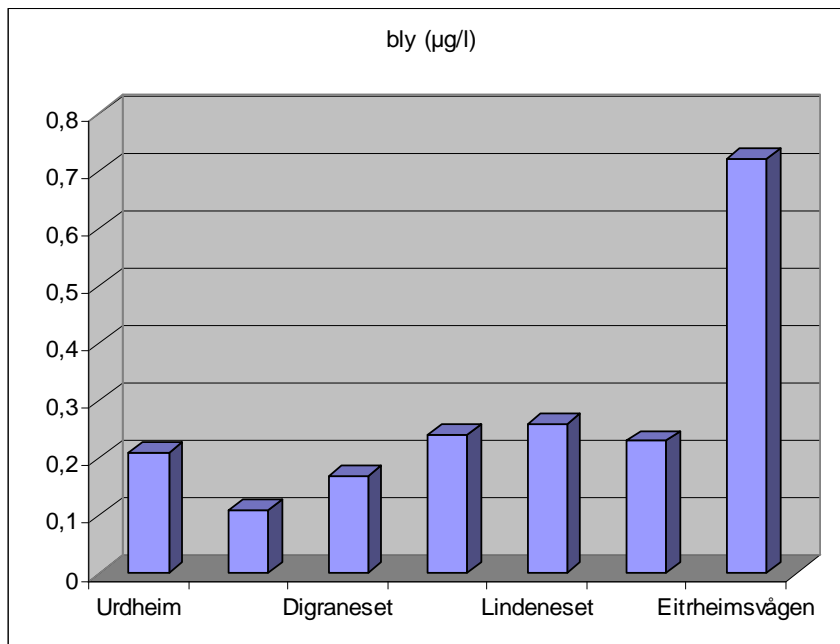
Figur 7. Konsentrasjonen av bly (µg/l) i overflatevann fra innerst (høyre) til ytterst (venstre) i Sjørfjorden i 2009 (årgjennomsnitt).
