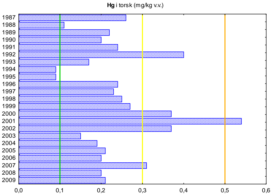
Figur 10. Gjennomsnittsverdier av kvikksølv i muskel av torsk fra indre Sør fjorden (1987-2009), mg/kg våtvekt. Verdiene er også gjengitt i Tabell 4. Nedre grenser for Klifs tilstandsklasser for miljøkvalitet er angitt; grønn: Kl. II (moderat forurenset); gul: Kl. III (markert forurenset); oransje: Kl. IV (sterkt forurenset); rød: Kl. V (meget sterkt forurenset).
